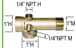
Conexión de 5 vías en bronce 1" 110 mm de largo
